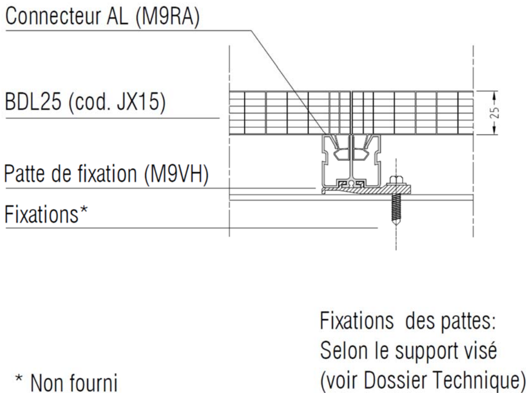
Figure 40– Support intermédiaire - Pose avec point fixe haut
