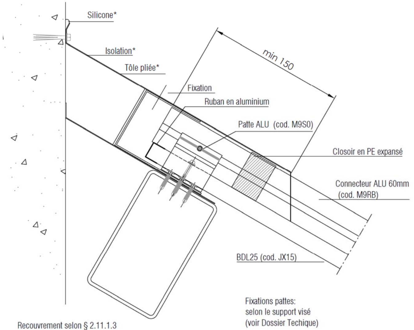
Figure 27I – Faîtage solin avec point fixe haut et connecteur M9RB
