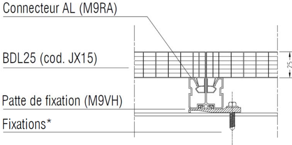
Figure 30 – Support intermédiaire - Pose avec point fixe bas
